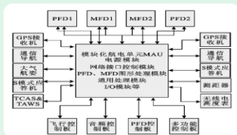
航电模块接口图
