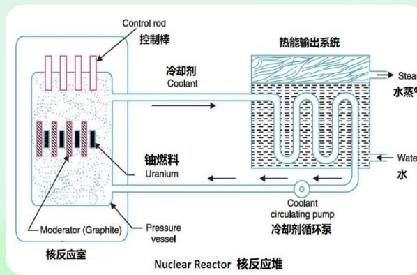
反应堆冷却系统
