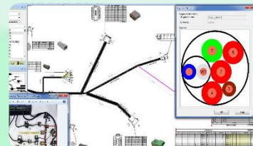
线缆连接图 / 线束图
