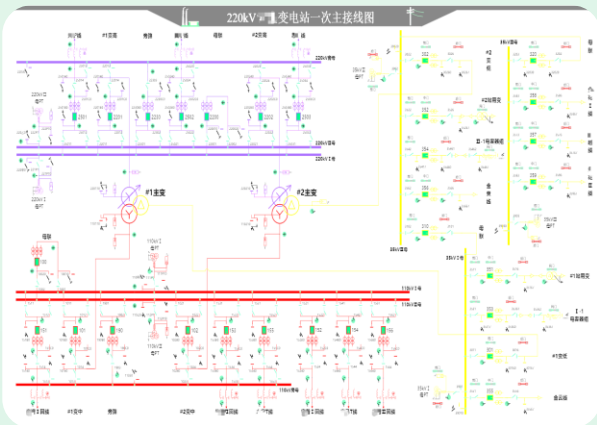
变电站接线图、电路图
