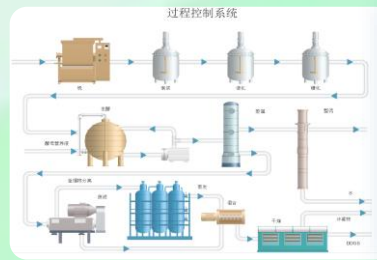
过程控制图、管道运输图
