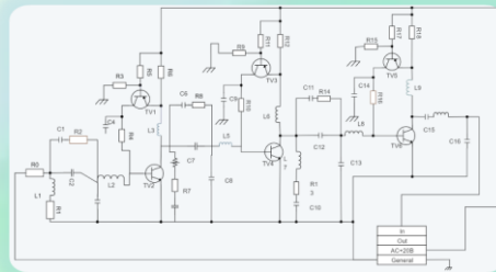
集成电路图
