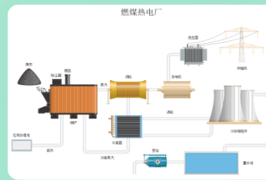
工艺流程图
